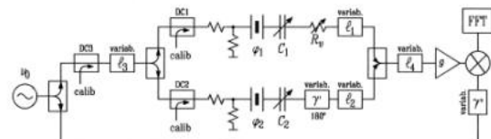
Figure 2. – Principe du banc de mesure LPMO.
