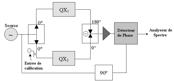
Figure 1. – Principe du banc de mesure CR200A.
